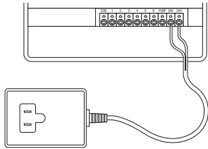
FIGURA 16: Collegamento del trasformatore
