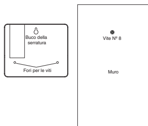
FIGURA 15: Installazione di un timer per interni
