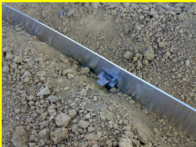
Bordura in alluminio altezza 11 cm
